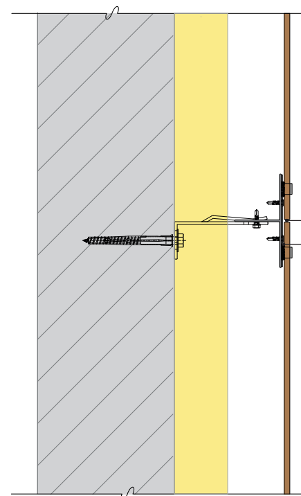
HORIZONTAL SECTION DETAIL / DETALLE SECCIÓN HORIZONTAL
