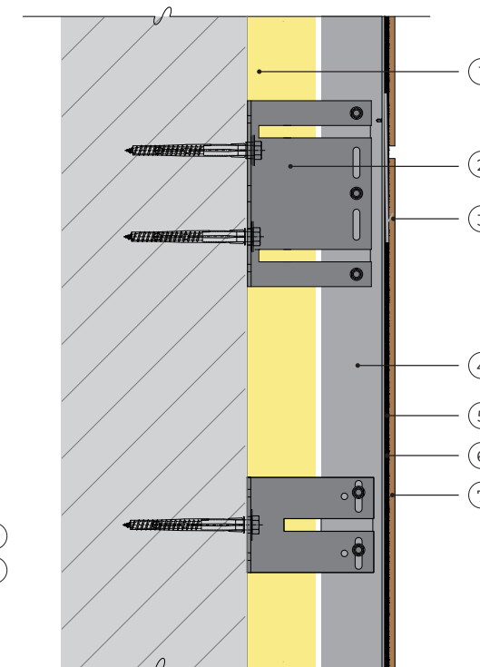
VERTICAL SECTION DETAIL / DETALLE SECCIÓN VERTICAL
